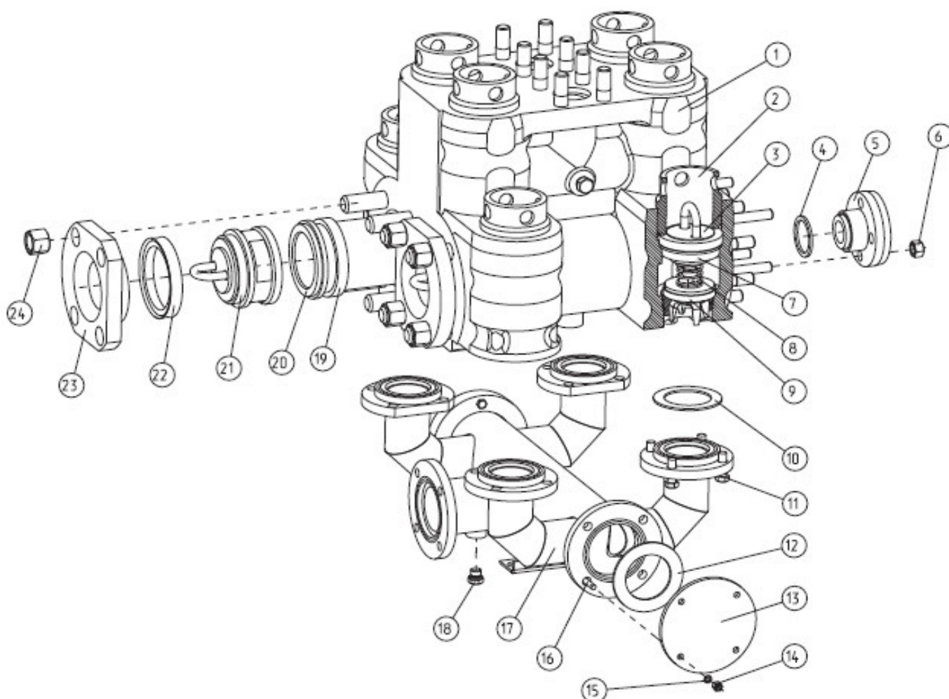
Гидравлическая часть АФНИ.306555.001-02
