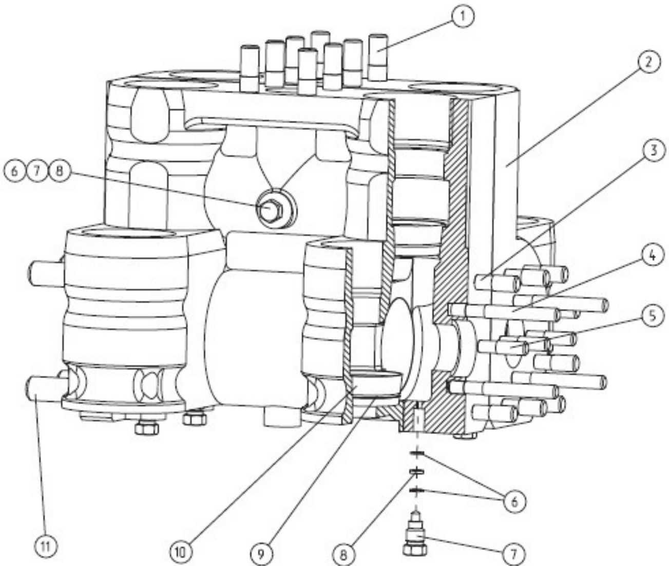
Блок клапанных коробок АФНИ.306555.002
